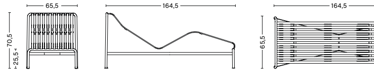
PALISSADE CHAISE LONGUE WIDTH 65,5 CM DEPTH 164,5 CM HEIGHT 70,5 CM SEAT HEIGHT 25,5 CM
